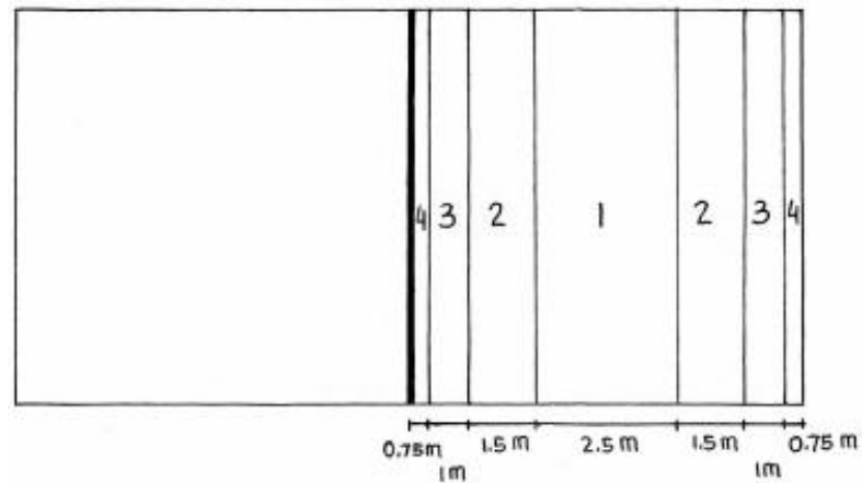
Gambar 4: Lapangan Tes Blok (Sumber: Furkon & Shandi, 2019)
